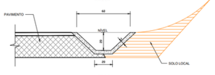
SARJETAS TRAPEZOIDAIS DE CONCRETO E GRAMA
