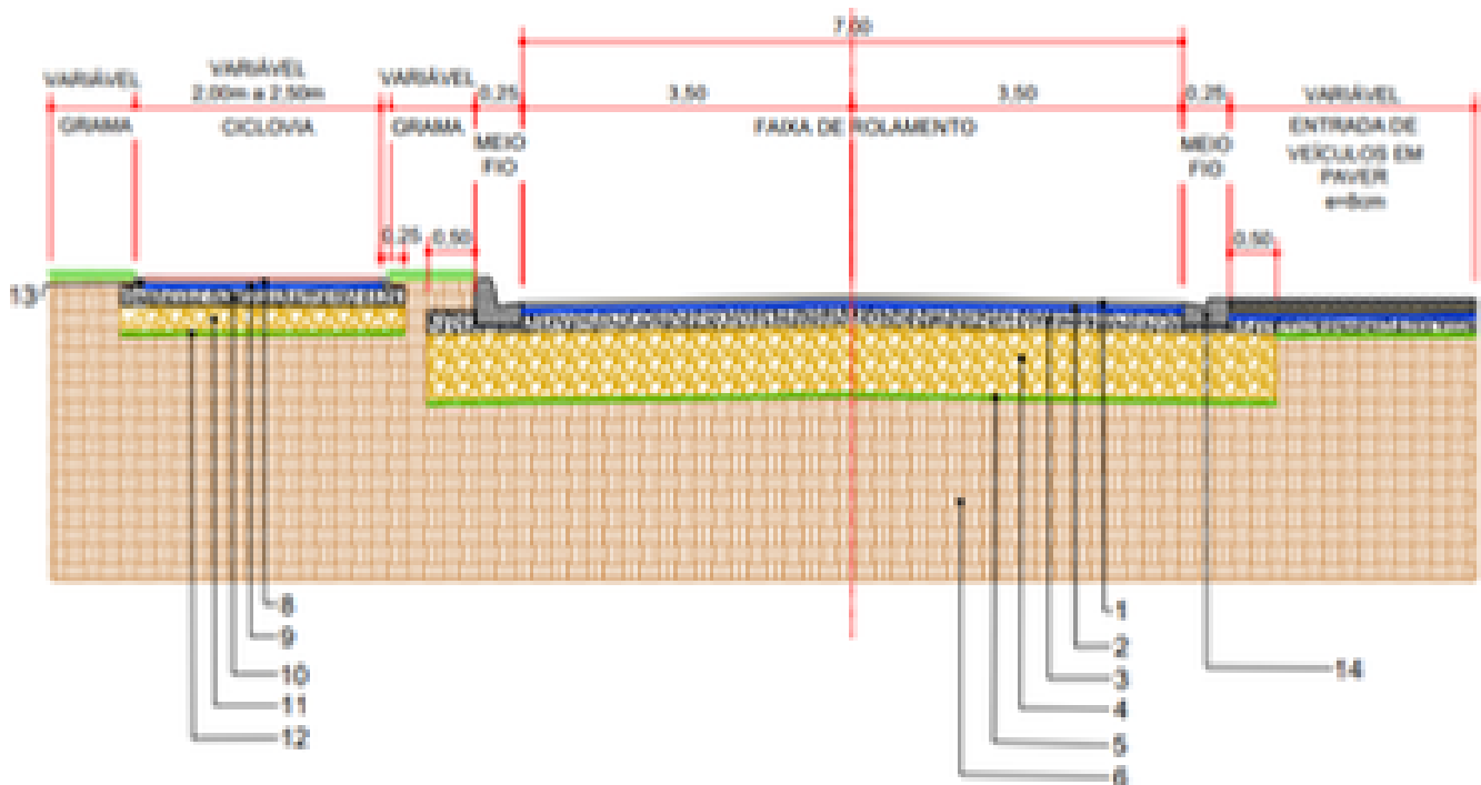
SEÇÃO TIPO 01 - ALARGAMENTO
